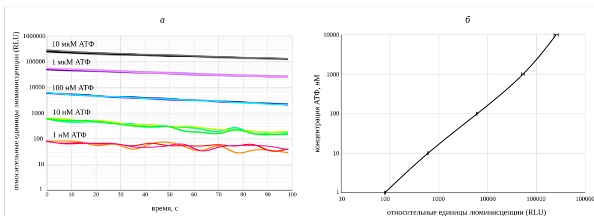
Рис. П1. Градуировочная зависимость биолуминесцентного сигнала от концентрации АТФ. а – Зависимость люминесценции (выраженной в относительных единицах RLU, по оси ординат в логарифмических координатах) от времени в присутствии АТФ в различных концентрациях. б – Градуировочная зависимость, построенная по усреднённым значениям люминесценции в начальный 5 с интервал времени
